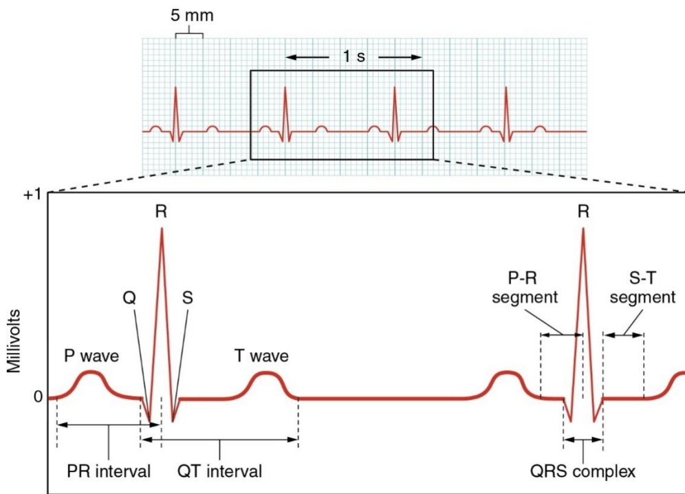
6.1. attēls. Elektrokardiogramma [41]
