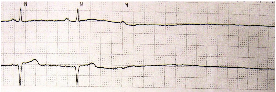
6.3. attēls. Asistolija
